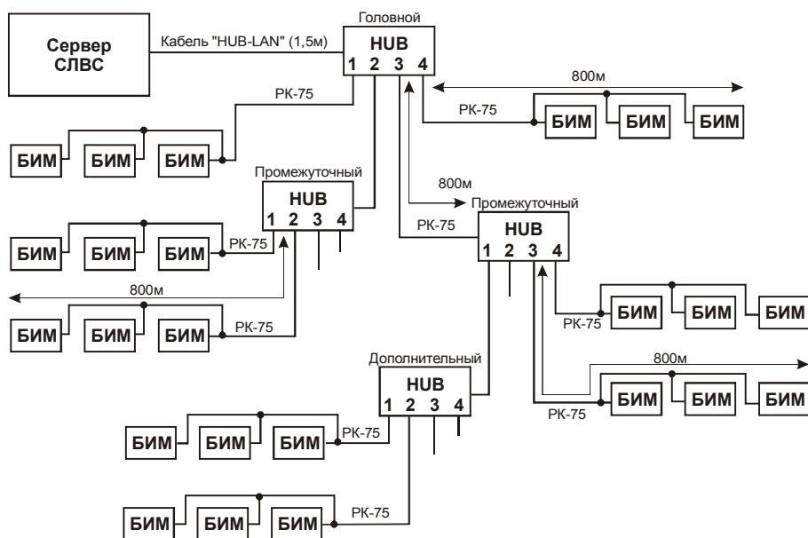
Рис. 3 Разветвленная сеть.
