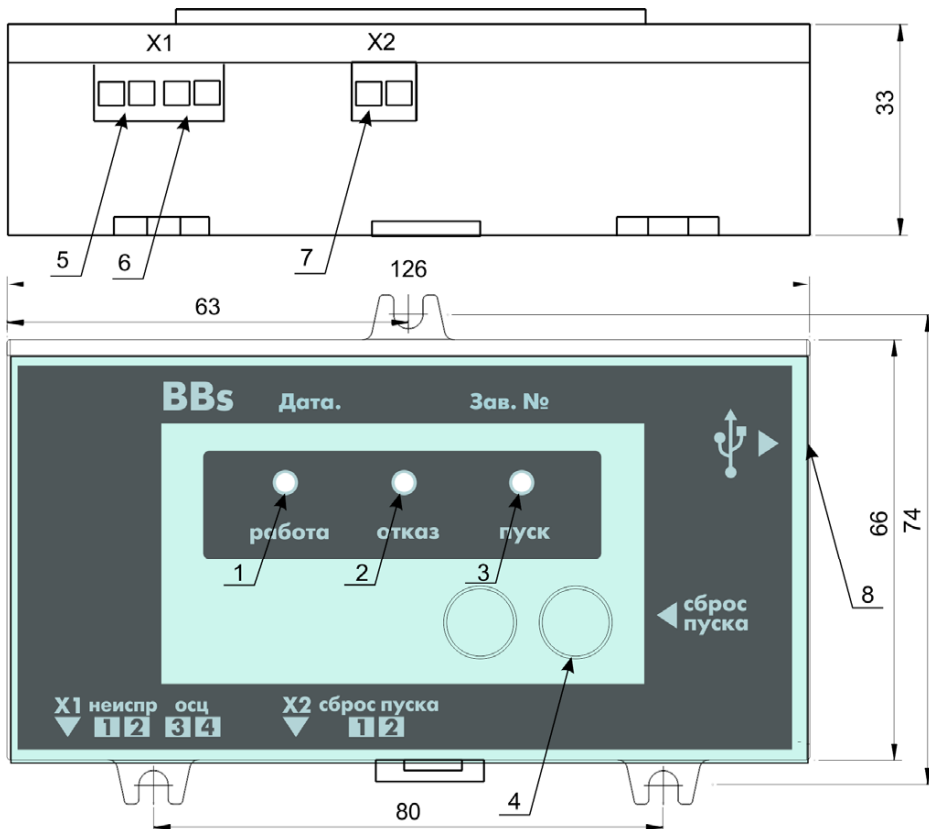
Рис. 1. Блок сигнализации ВВs
