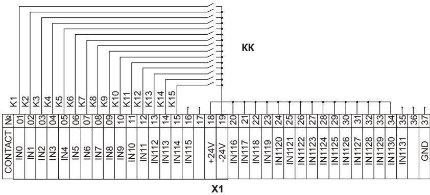
Рис. 2. Ввод дискретных каналов (кабель КД1)
