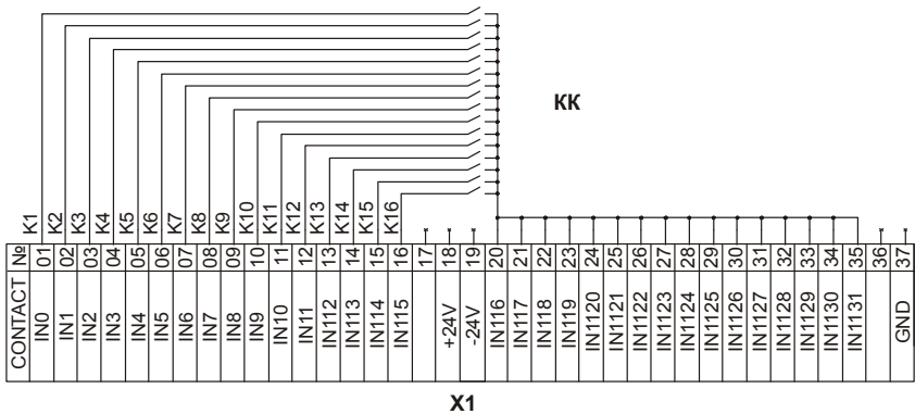
Рис. 3 Ввод дискретных каналов (кабель КД2)
