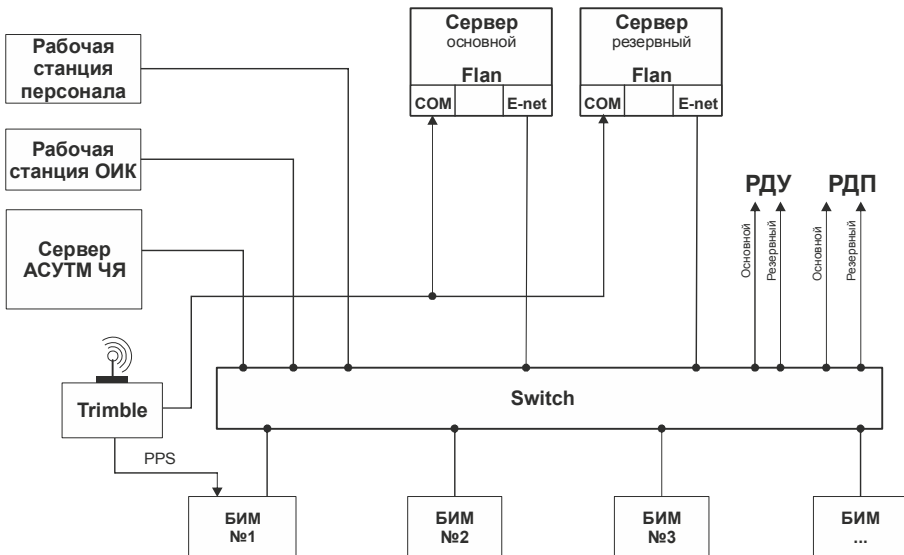
Рис. 2 Комплекс ЧЯ в сети Ethernet.
