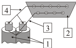
Рис. 6. Монтаж кабеля линии ЛВС с разъемами DB-9
