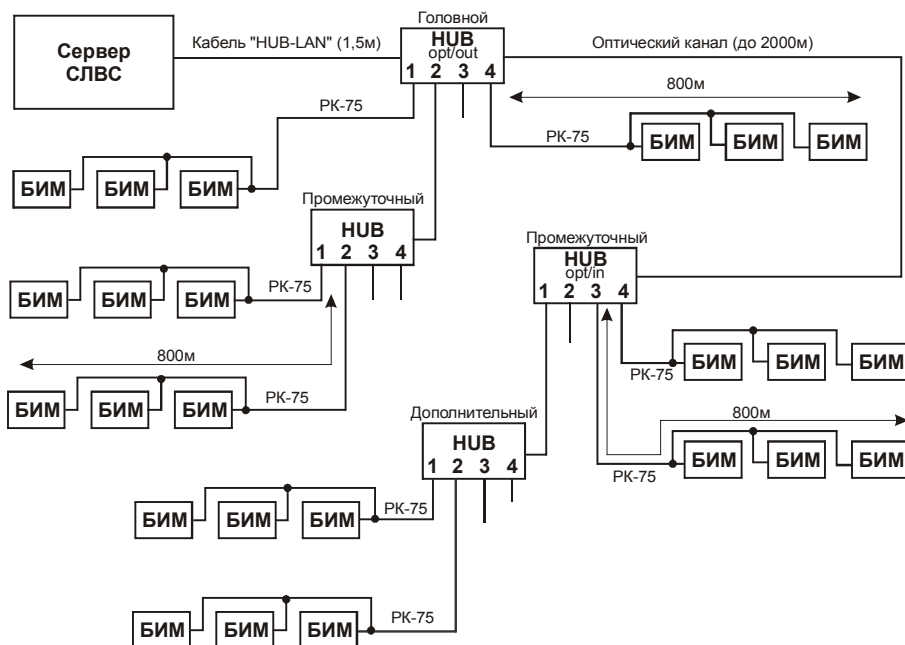
Рис. 4 Схема подключения оптической линии связи.
