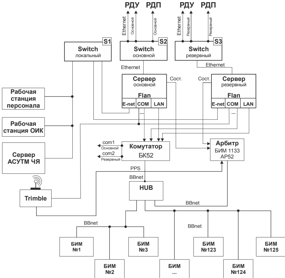
Рис. 5 Резервирование сервера в СЛВС ЧЯ.
