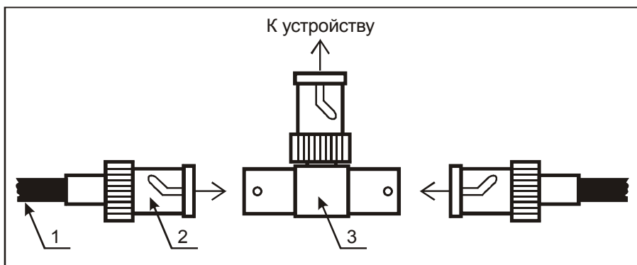
Рис. 7. Подключение разъемов BNC. 1 – кабель РК-75 RG-6; 2 – BNC разъем на кабель; 3 – Т-образный тройник;
