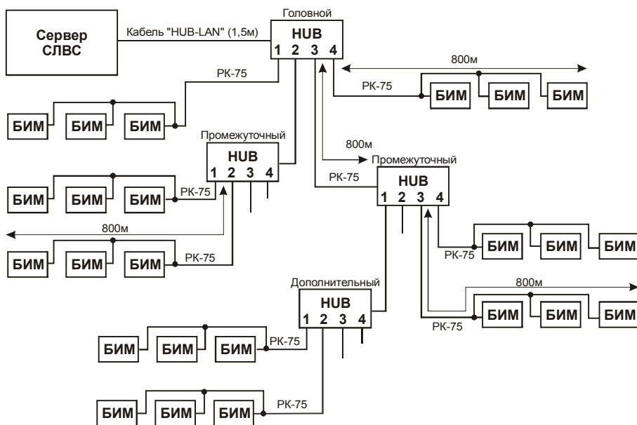
Рис. 3 Разветвленная сеть.
