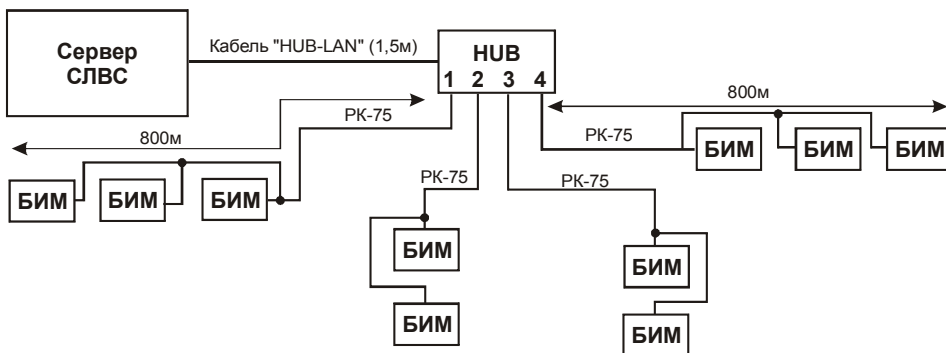
Рис. 1 Структурная схема участка СЛВС ЧЯ.
