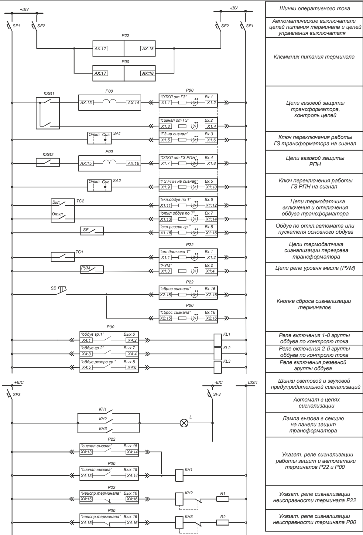
Рис. 50 Схема подключения цепей питания, управления, блокировок, сигнализации
