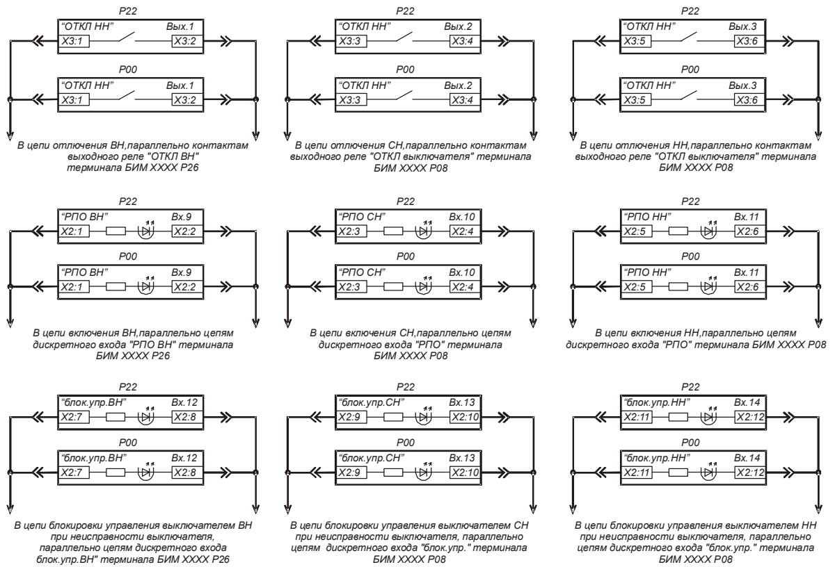
Рис. 48 Схема подключения цепей отключения выключателей VН, СН, и НН
