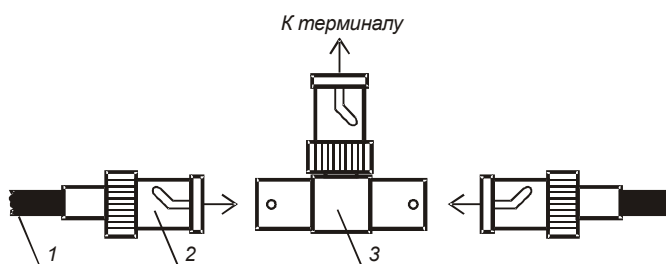
Рис. 9 Подключение разъемов BNC
