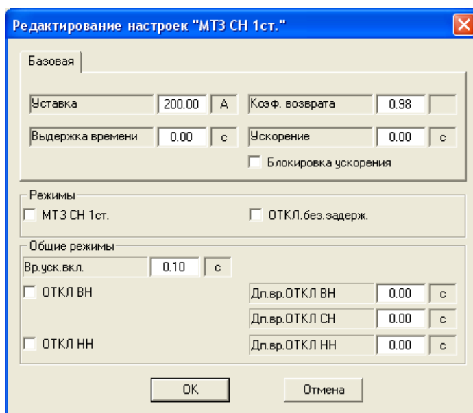
Рис. 22 Редактор настроек «МТЗ СН 1 ст.»
