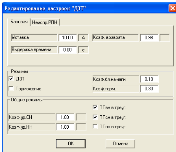
Рис. 19 Редактор настроек «ДЗТ»
