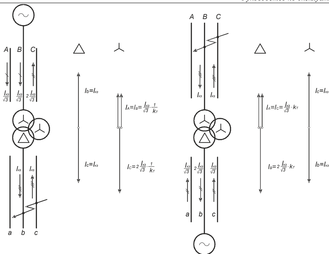
Рис. 35 Диаграммы подключения токов на аналоговые входы терминалов для проверки ДЗТ и ДО
