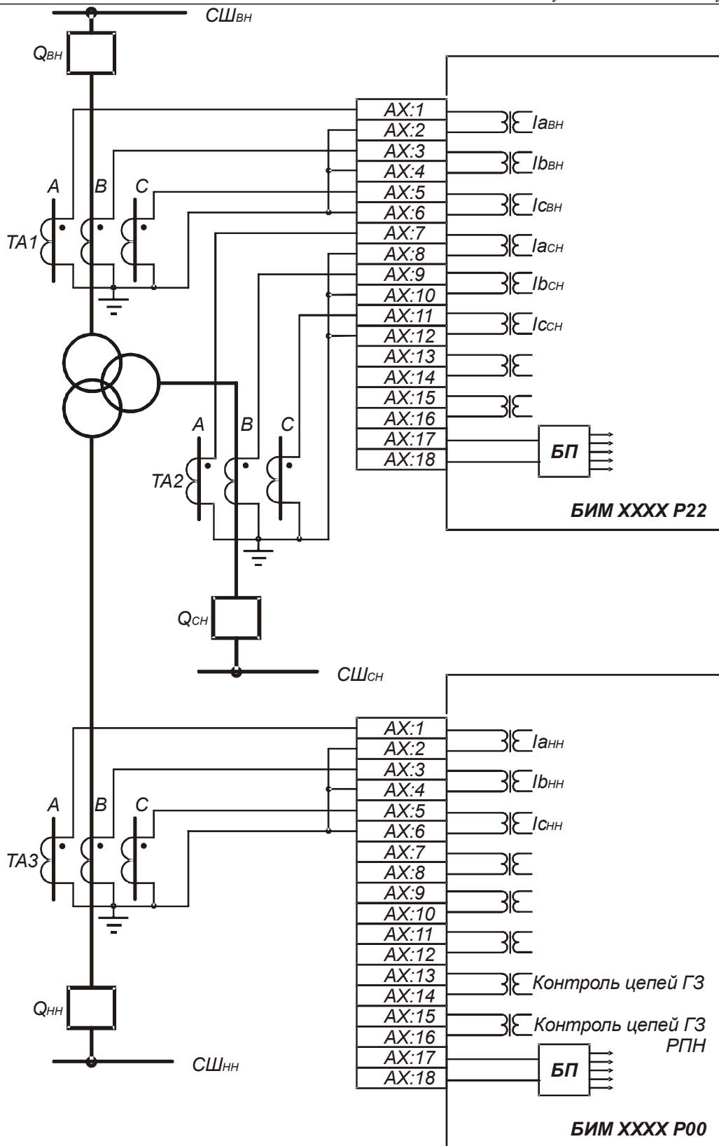
Рис. 51 Схема подключения аналоговых цепей
