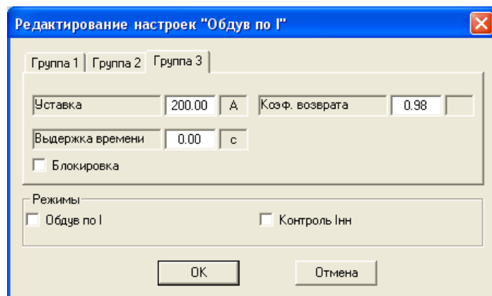
Рис. 23 Редактор настроек «Обдув по I»
