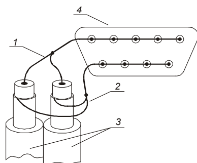
Рис. 8 Подключение кабелей RG-6 к разъёму DB-9F
