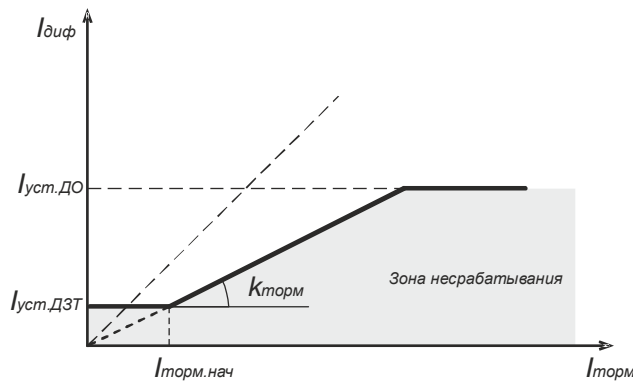
Рис. 6 Тормозная характеристика ДЗТ
