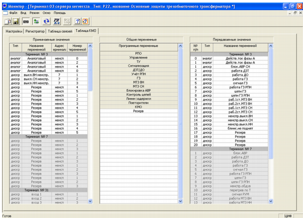
Рис. 15 Страница «Таблица КМО»
