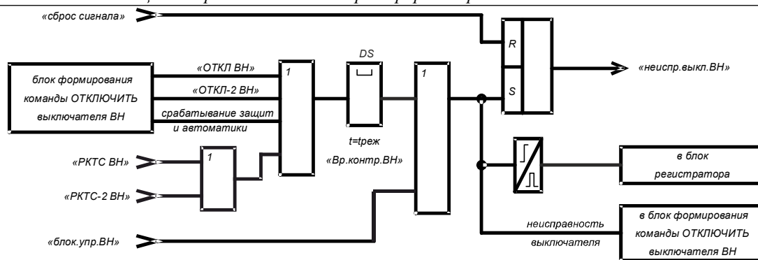
Рис. 43 Функциональная схема блока контроля цепей управления выключателя ВН
