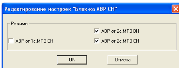
Рис. 25 Редактор настроек «Блок-ка АВР СН» в терминале P22
