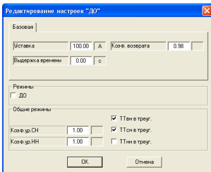
Рис. 21 Редактор настроек «ДО»
