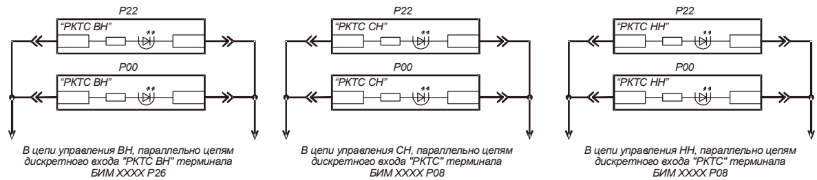
Рис. 49 Схема подключения РКТС
