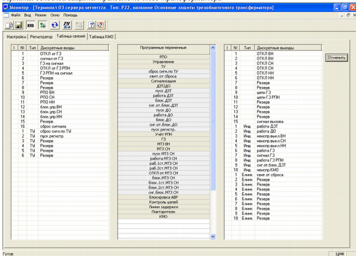
Рис. 13 Страница «Таблица связей»
